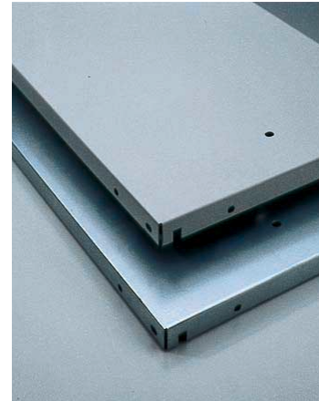
Fachboden mit Abkantung 25 mm. Optimiert für den Ordneinsatz.
