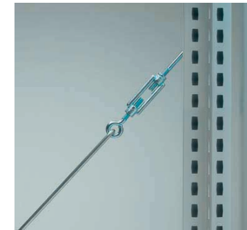
Fachbodenträger und Fachböden einfach stecken, Diagonalversteifung spannen, fertig! Alles ohne Werkzeug!
